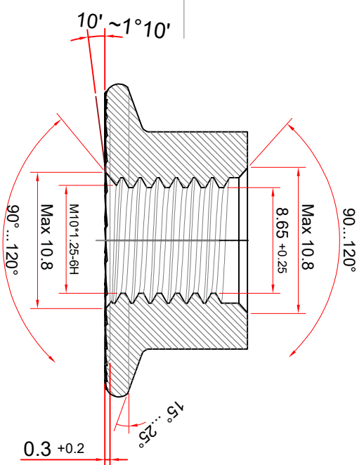
SECTION A-A scale : 2.4 : 1
