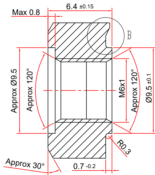
SECTION A-A SCALE 4:1
